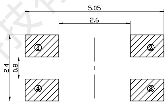
安装参考图
